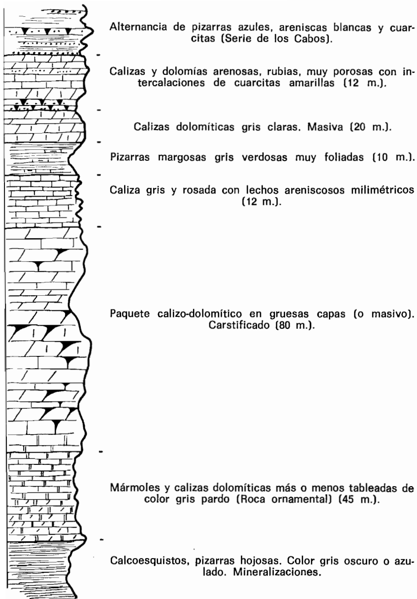
SERIE DE LA CALIZA DE VEGADEO SECTOR DE SEOANE DEL CAUREL
