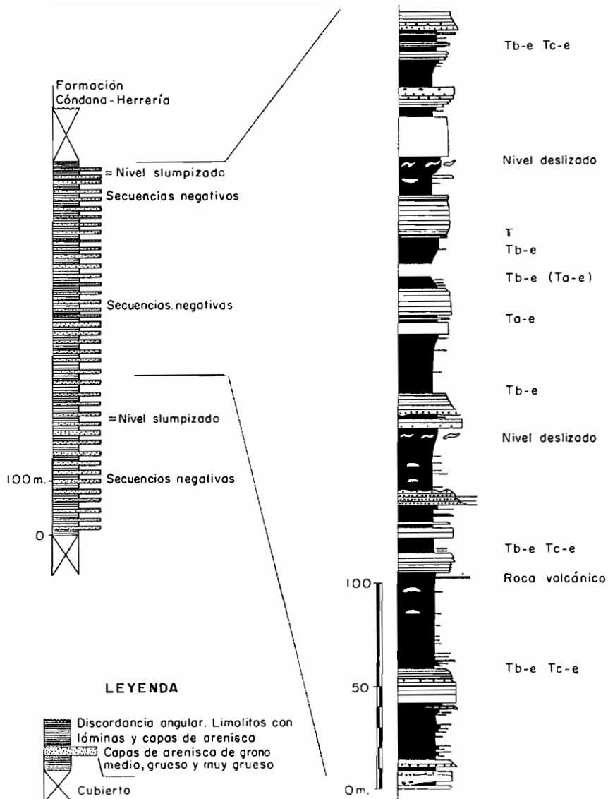
COLUMNA PARCIAL DEL PRECAMBRICO AL N. DE LA FALLA DE CORNOMBRE- LA URZ. CAMINO DEL VALLE GRANDE DE SALCE.
