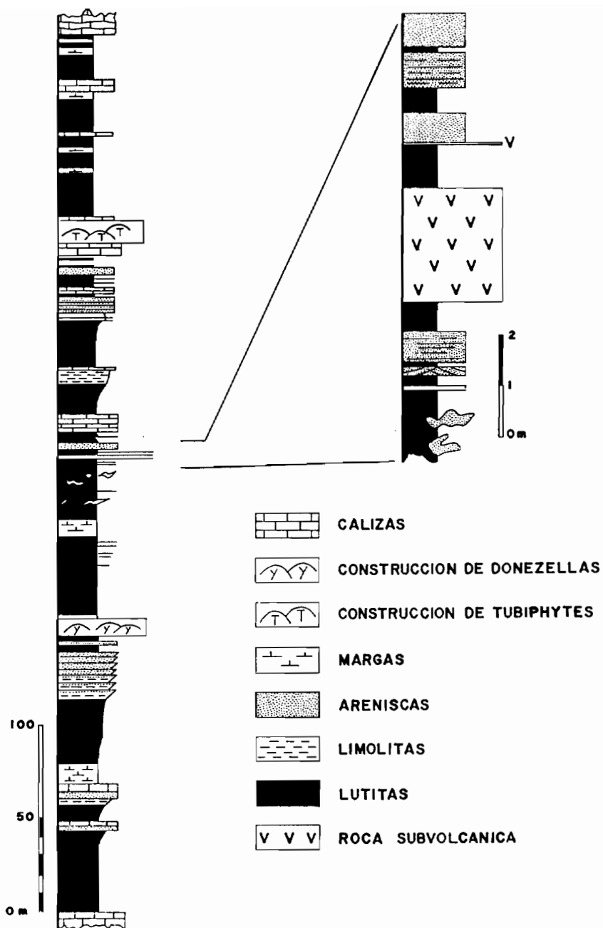
Figura 8. Columna estratigráfica esquemática de la Formación San Emilianense en la sección de Villafeliz (Manto de Bodón).
