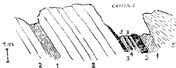
Figura 5.—Corte del yacimiento de hematites de la «Casa del Coxu» (Ordovaga): 1 y 4. Pizarras azuladas; 2. Cuarzitas; 3. Hematites-oligistas; 5. Pizarras abigarradas. Según LLOPIS (1961).
