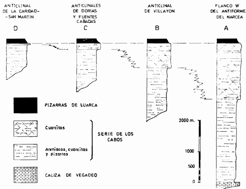
Figura 2.—Sucesión estratigráfica de la Serie de los Cabos en los diferentes afloramientos existentes en la Hoja. La disminución del espesor de los niveles superiores cuarcíticos de E a O destaca claramente.
