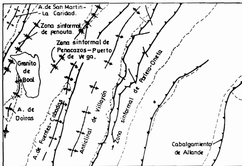
Figura 1.—Mapa con la posición de las estructuras mencionadas en el texto.
