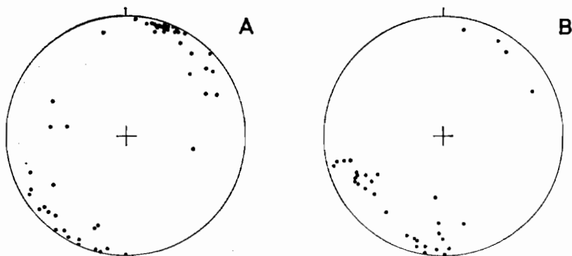
Figura 9.—Estereograma mostrando la disposición de los planos de diaclasas en los alrededores de Tapia de Casariego.
