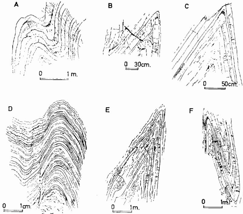
Figura 7. —Morfología de los pliegues de primera fase. A, pliegue aproximadamente concéntrico; B, C y E, pliegues tipo chevron; D, pliegue similar; F, pliegue similar, fuertemente aplastado. Corte de la costa en los alrededores de Tapiá de Casariego (Serie de los Cabos).
