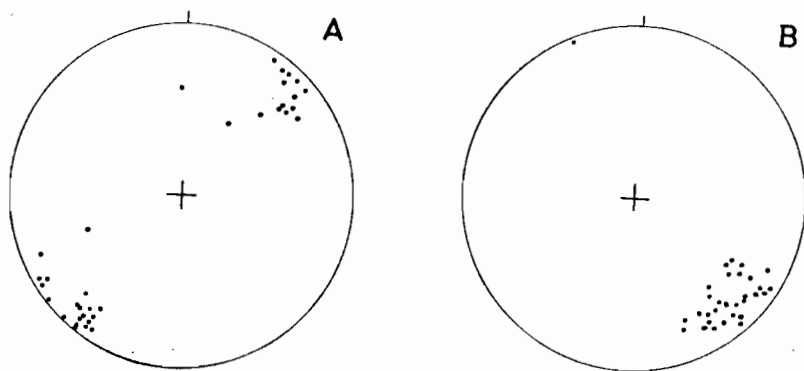
Figura 6.—Estereogramas mostrando la disposición de los ejes (A) y superficies axiales (B) de los pliegues menores de primera fase. Corte de la costa en los alrededores de Tapia de Casariego.
