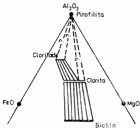
Figura 10.—Representación AFM de las paragénesis por encima de la isograda de la biotita o cloritoide. Ambos minerales son incompatibles en una misma asociación.
