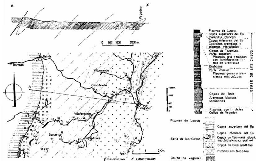
Figura 2.—Sucesión estratigráfica de la Serie de los Cabos al O de Vegadeo (según MARCOS et al., in litt.).
