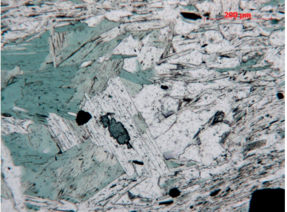
Figura 61. Ejemplo de esquivo claro de la Unidad de Calar Alto con dominios lenticulares ricos en moscovita y clorita con pequeños restos muy corroídos de cloritoide
