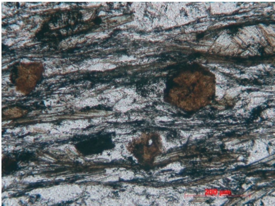
Figura 59. Muestra de esquistos grafitosos con oxiclорitas pseudomorfizando a granates. Además se observan dominios lenticulares previos a la formación principal ricos en clorita. Esquistos grafitosos (1) de la Unidad de Calar Alto, Lomo de Bas
