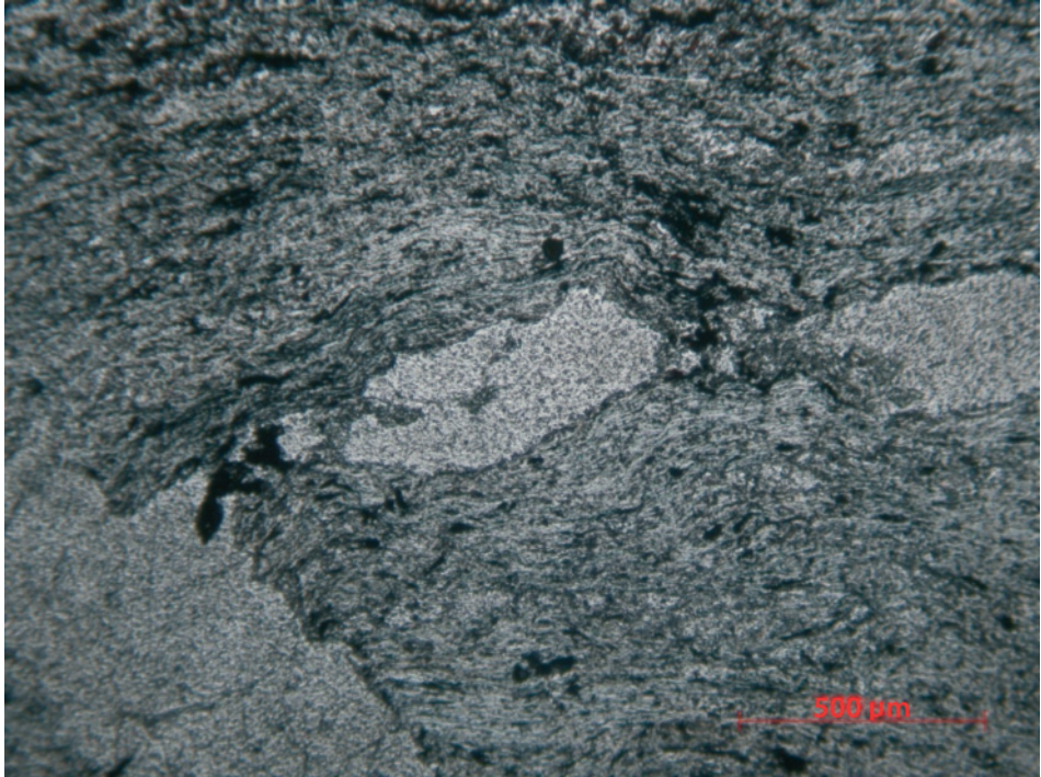
Figura 75. Lámina delgada de una filita de la imbricación inferior del Maláguide Inferior (22) caracterizada por una asociación mineral formada por illita+clorita+pirofilita, junto con cuarzo y calcita. En esta imagen se observan boudines de una vena de calcita
