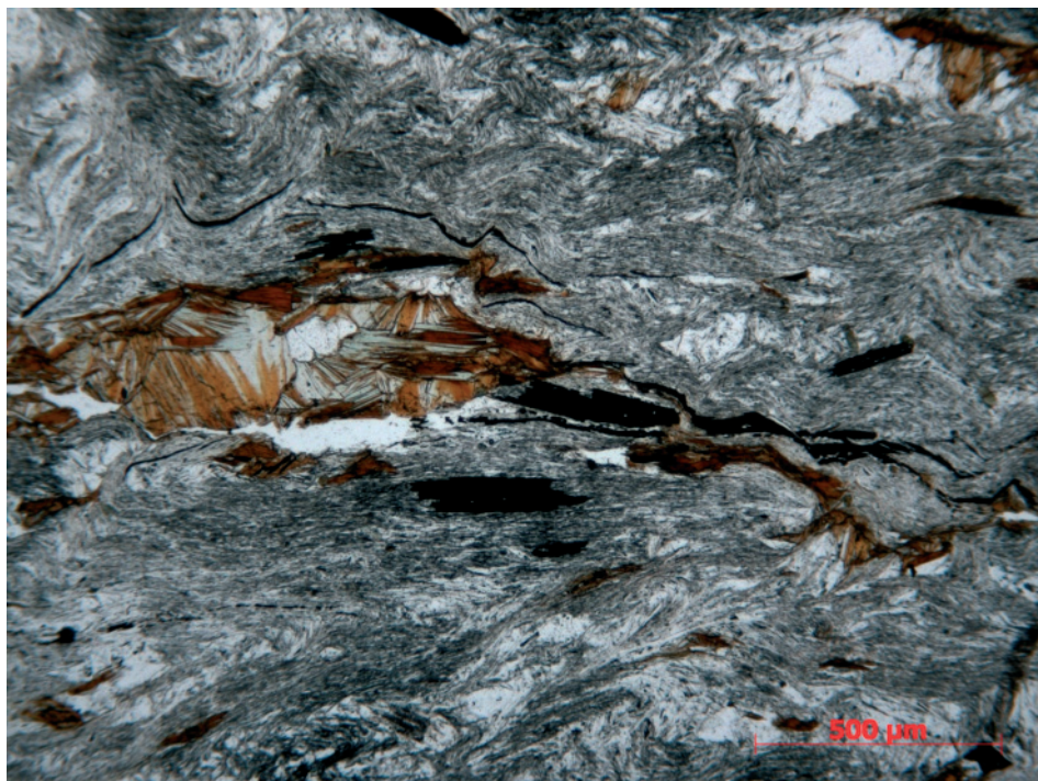
Figura 58. Muestra de esquistos grafitosos de la Unidad de Calar Alto con dominios lenticulares formados por cuarzo y clorita muy alterada a oxiclrita de color marrón. Además se observan porfidoblastos negros de óxidos de hierro, probablemente pseudomorfos de cloritoide
