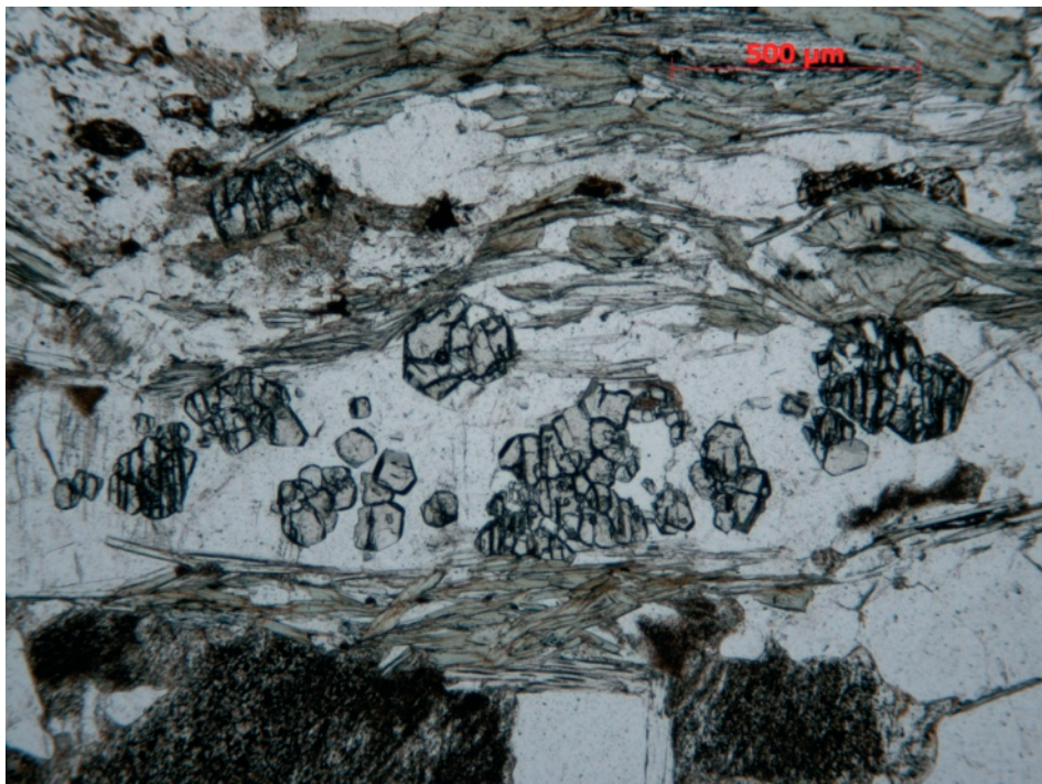
Figura 67. Lamina delgada de esquistu claro con granate, estaurolita y distena de la Unidad de Bédar-Macael (8). Además en esta foto se distingue abundante mica blanca, cuarzo y minerales accesorios como turmalina e ilmenita
