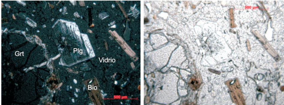
Figura 76. Muestra de dacita (43) del Puntarrón en la Hoja de Puerto Lumberas
