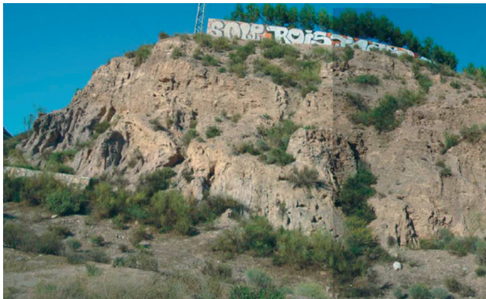
Figura 46. Conjunto sedimentario relacionado con la construcción de abanicos aluviales con progración proximal en onlap, correspondiente a la 2ª fase deposicional. Margen derecha de la rambla del Mundial 82. Hospital de Lorca al suroeste de la ciudad
