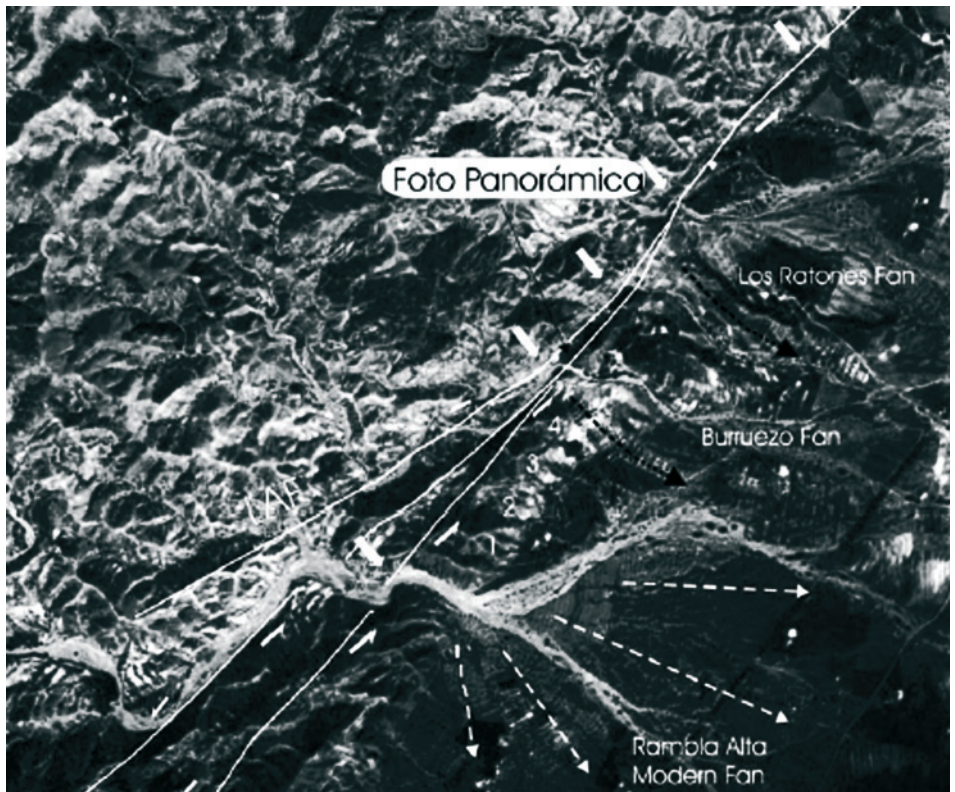
Figura 55. Foto aérea de la zona de falla de Lorca-Alhama de Murcia mostrando los desplazamientos sinistral y decapitaciones de ramblas (flechas blancas) que se registran entre Lorca y el Polígono Industrial de Rambla Alta. 1, 2, 3, 4, etc.; representan los lóbulos sedimentarios desplazados sinistralmente, correspondientes a la formación de Conglomerados de Rambla
