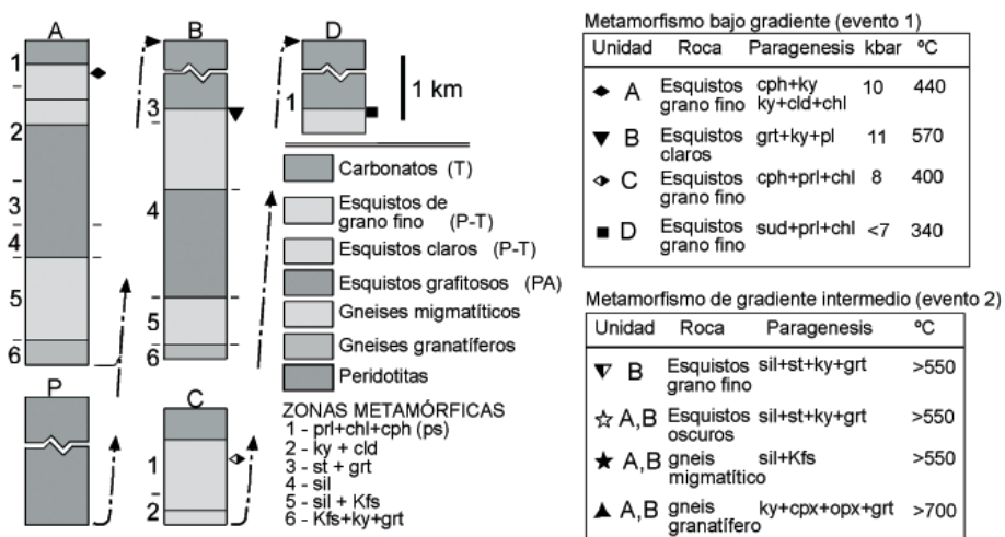
Figura 5. Secuencias litológicas y zonación metamórfica de las Unidades Alpujarrides aflorantes en las Béticas centrales y orientales, con su posición en la pila Alpujarride y las paragénesis minerales utilizadas para su distinción. Figura modificada de BALANYÁ et al. (1998)
